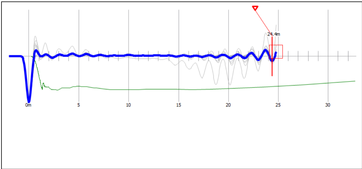
Reflectogram P-32
