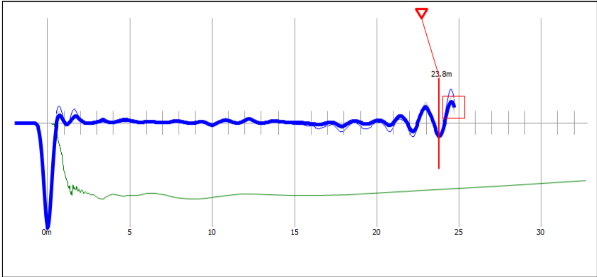
Reflectogram P-280
