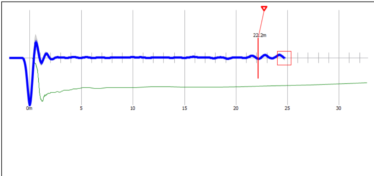
Reflectogram P-99
