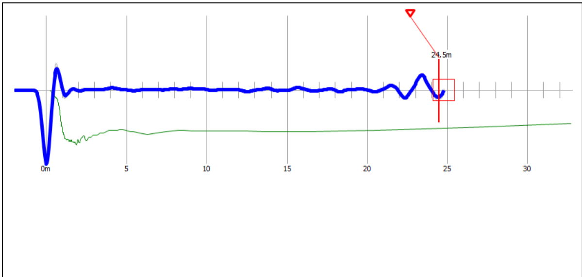
Reflectogram P-12
