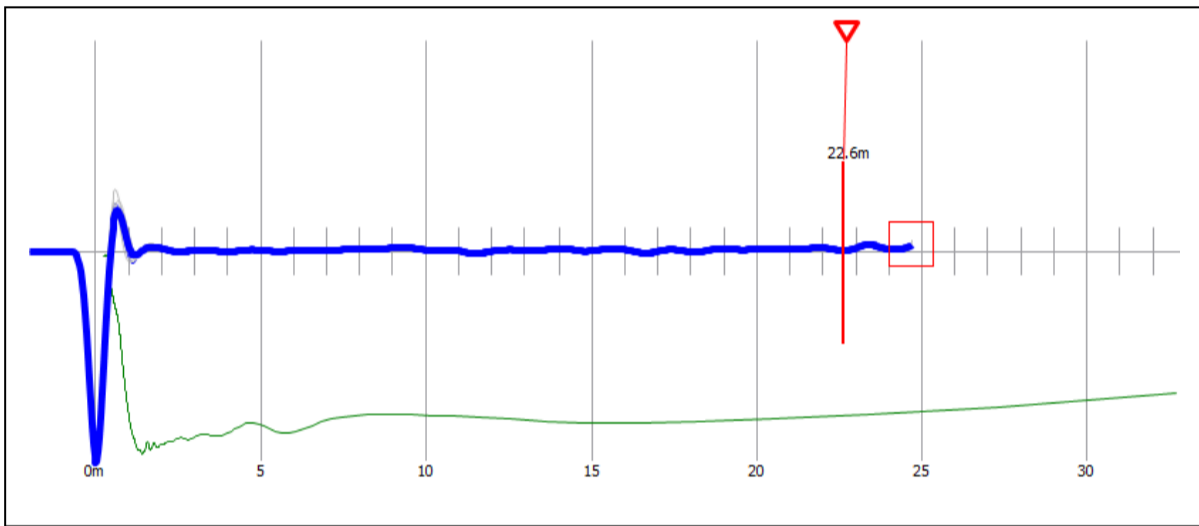
Reflectogram P-310
