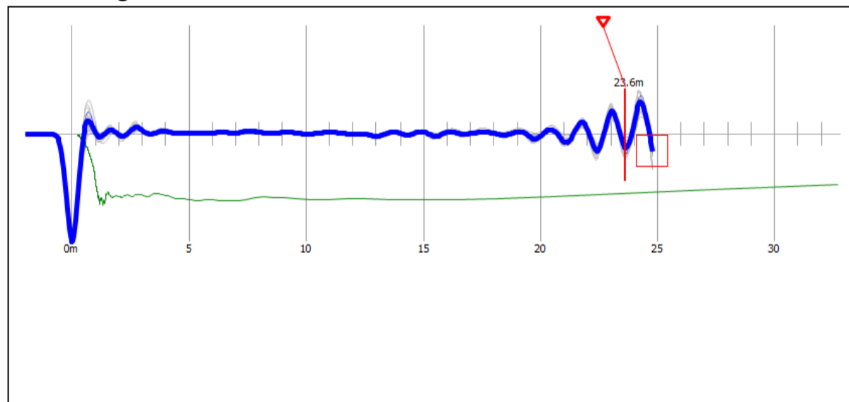
Reflectogram P-13
