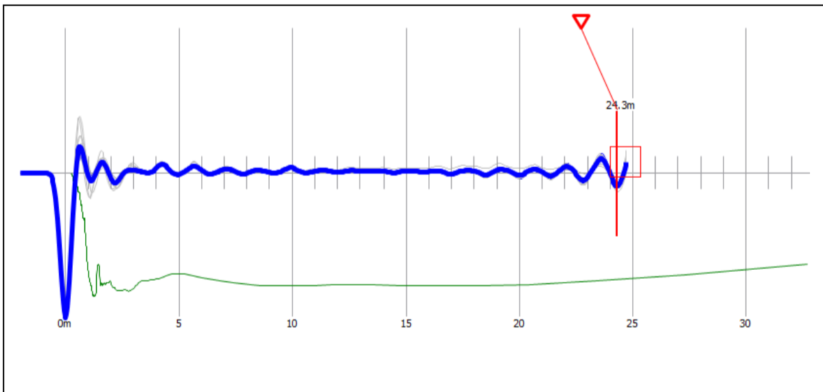
Reflectogram P-146
