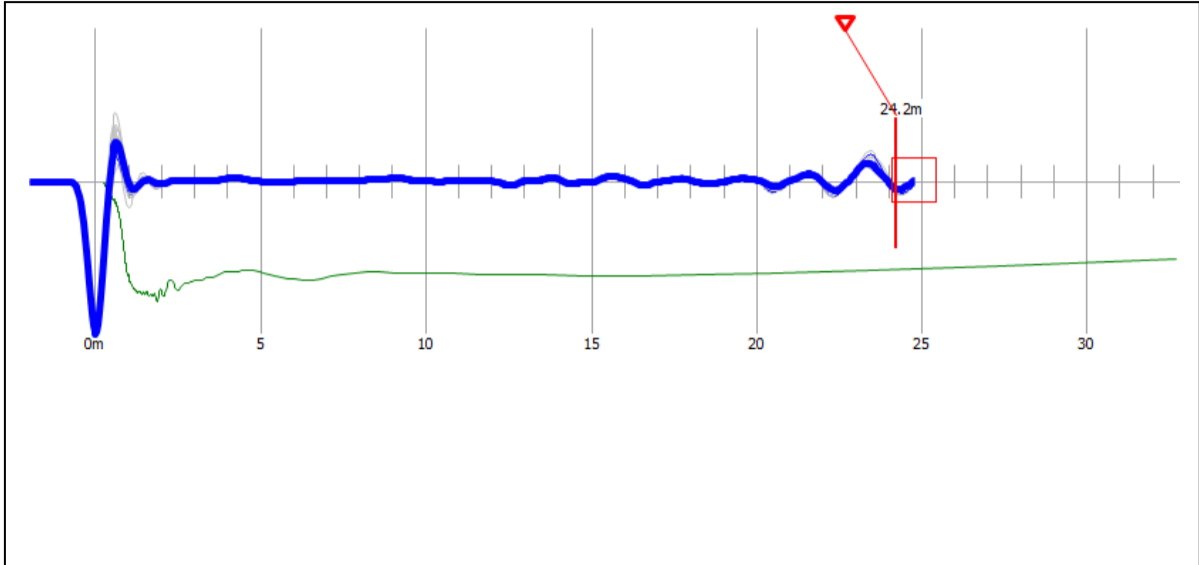
Reflectogram P-03
