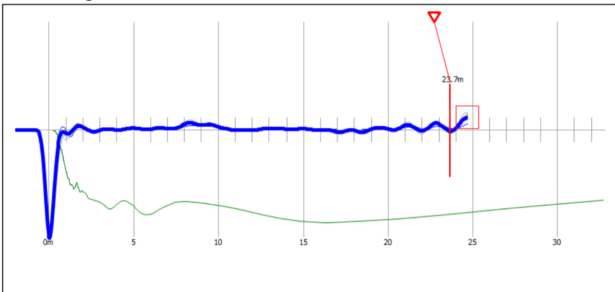
Reflectogram P-325
