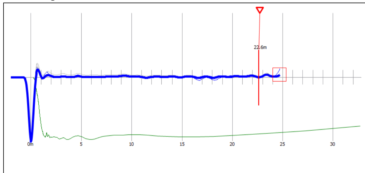
Reflectogram P-312
