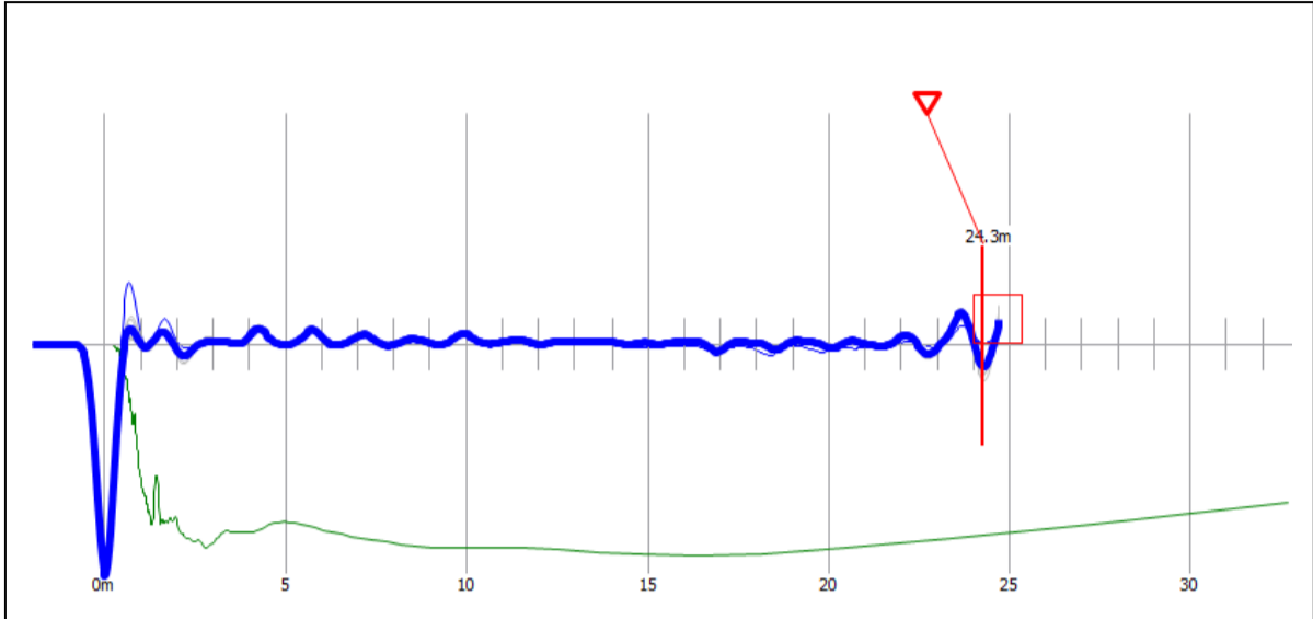
Reflectogram P-215
