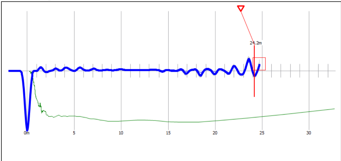
Reflectogram P-145
