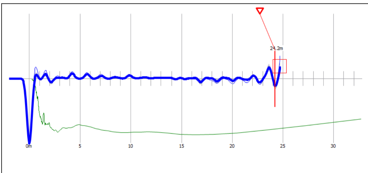
Reflectogram P-197
