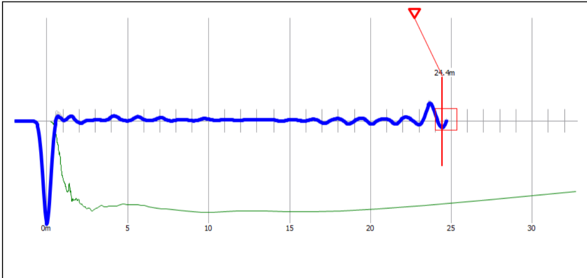
Reflectogram P-222
