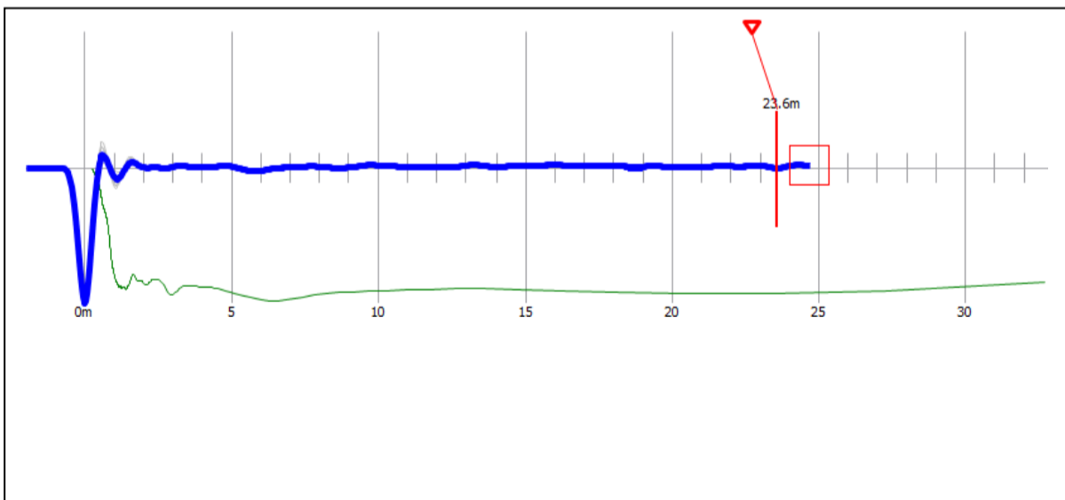
Reflectogram P-109
