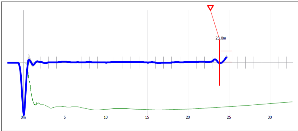
Reflectogram P-255
