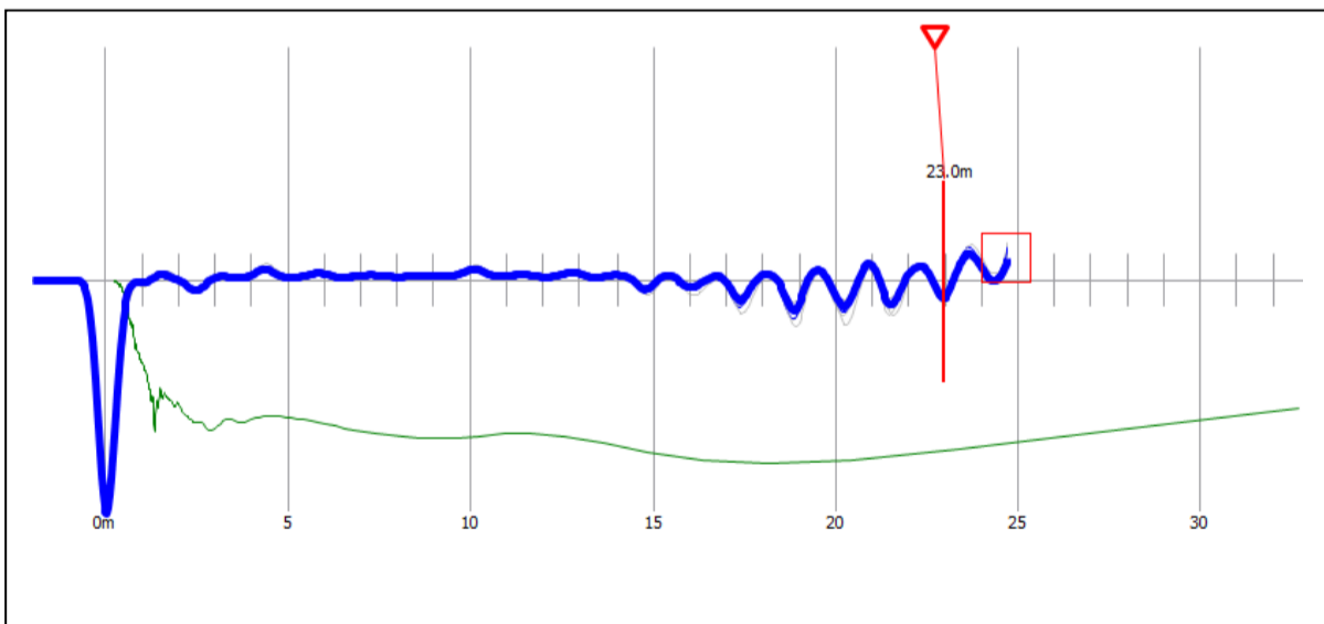
Reflectogram P-160
