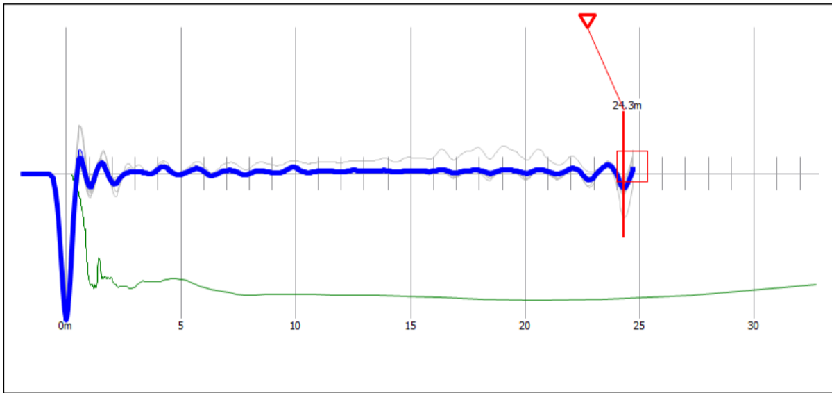
Reflectogram P-146
