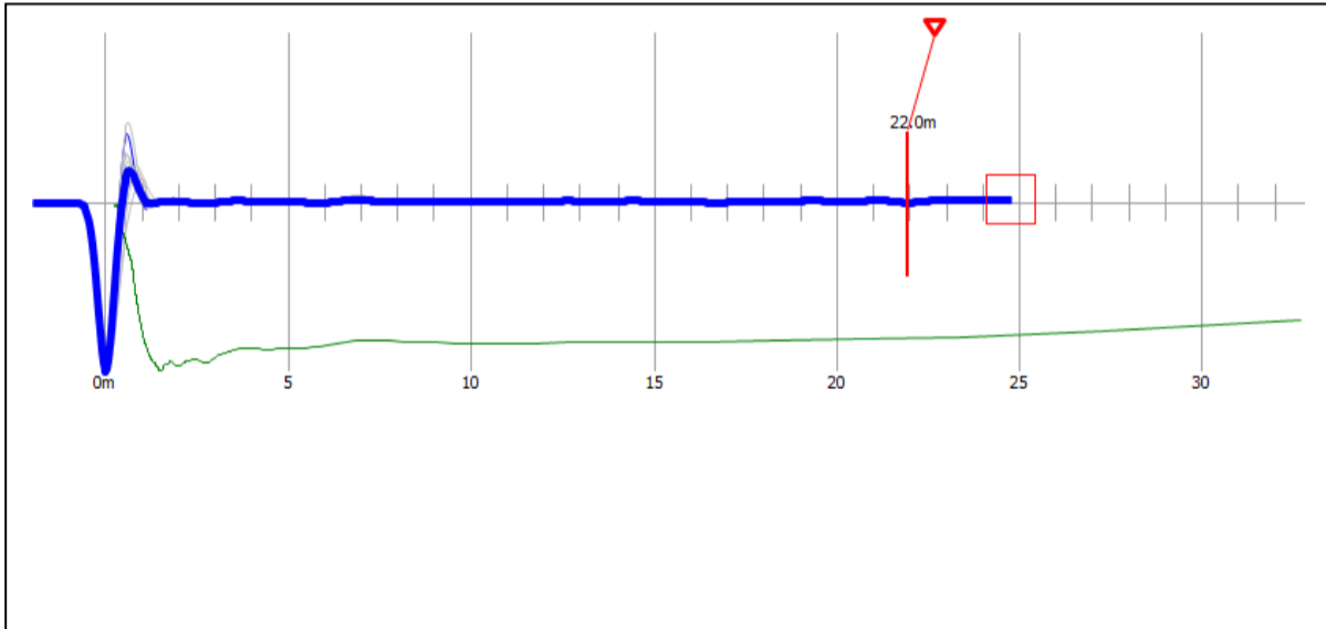
Reflectogram P-04
