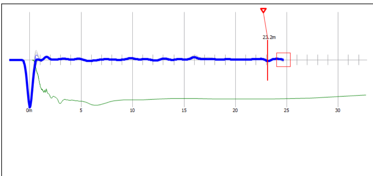
Reflectogram P-99
