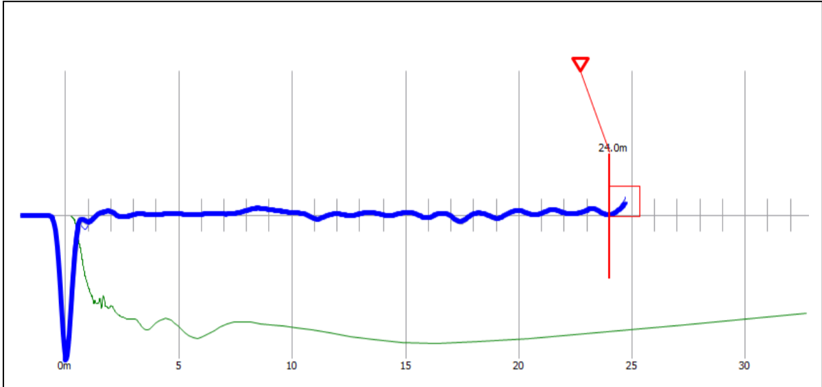
Reflectogram P-132
