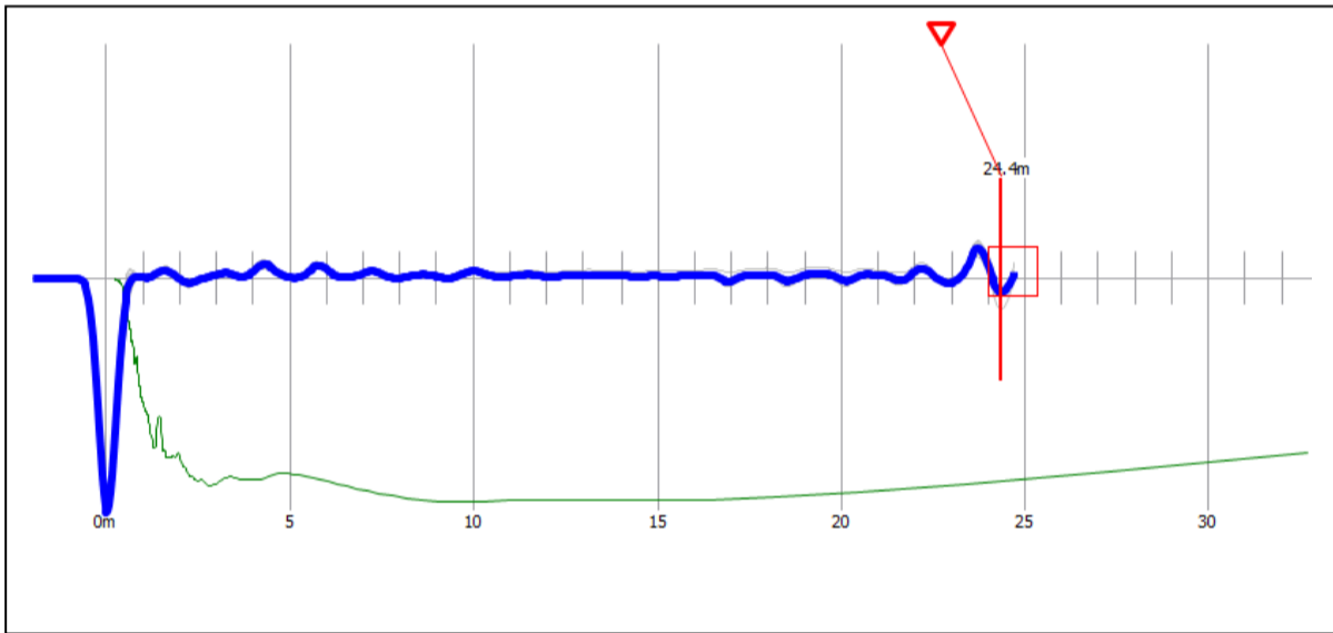
Reflectogram P-197
