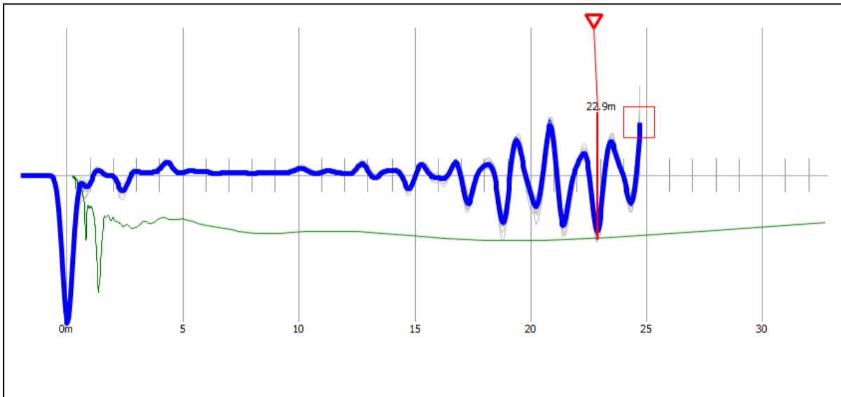
Reflectogram P-160
