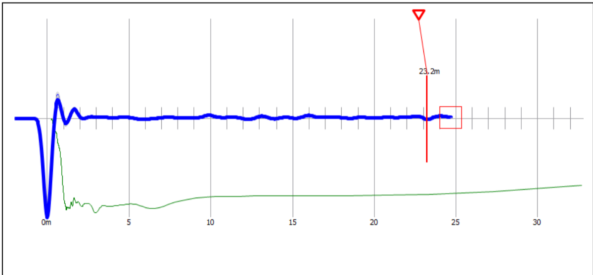
Reflectogram P-102
