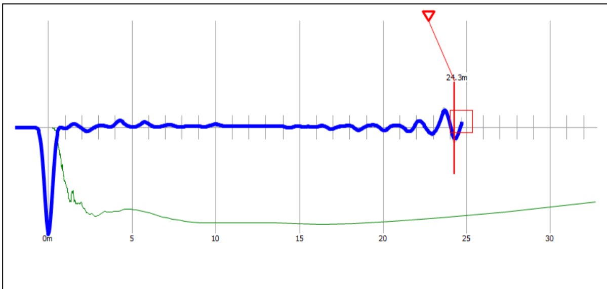
Reflectogram P-244
