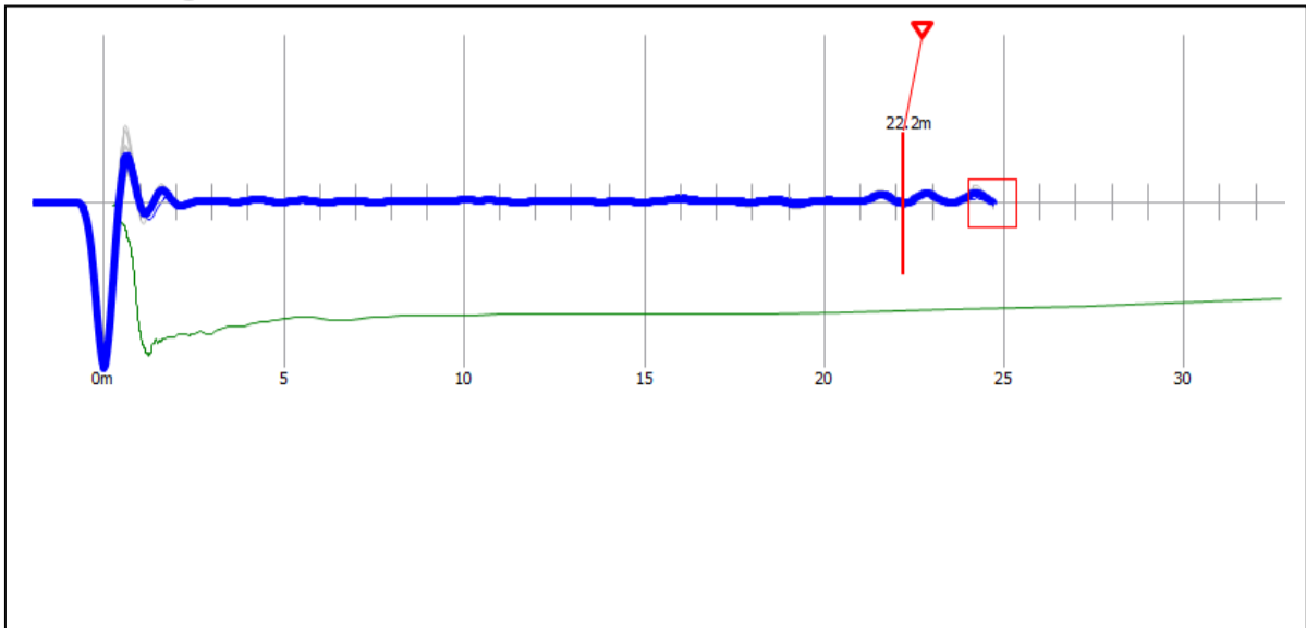
Reflectogram P-95
