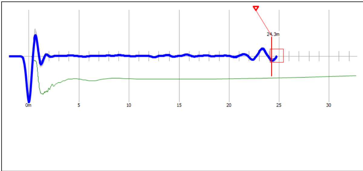
Reflectogram P-9
