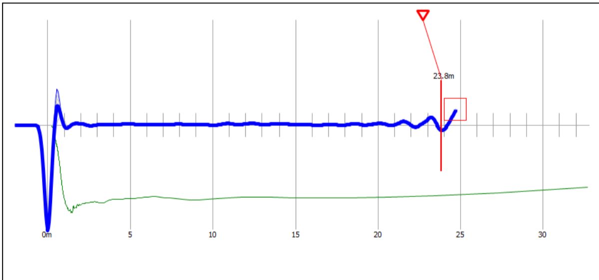
Reflectogram P-284
