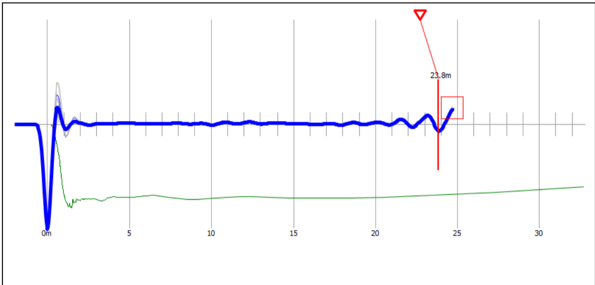
Reflectogram P-255
