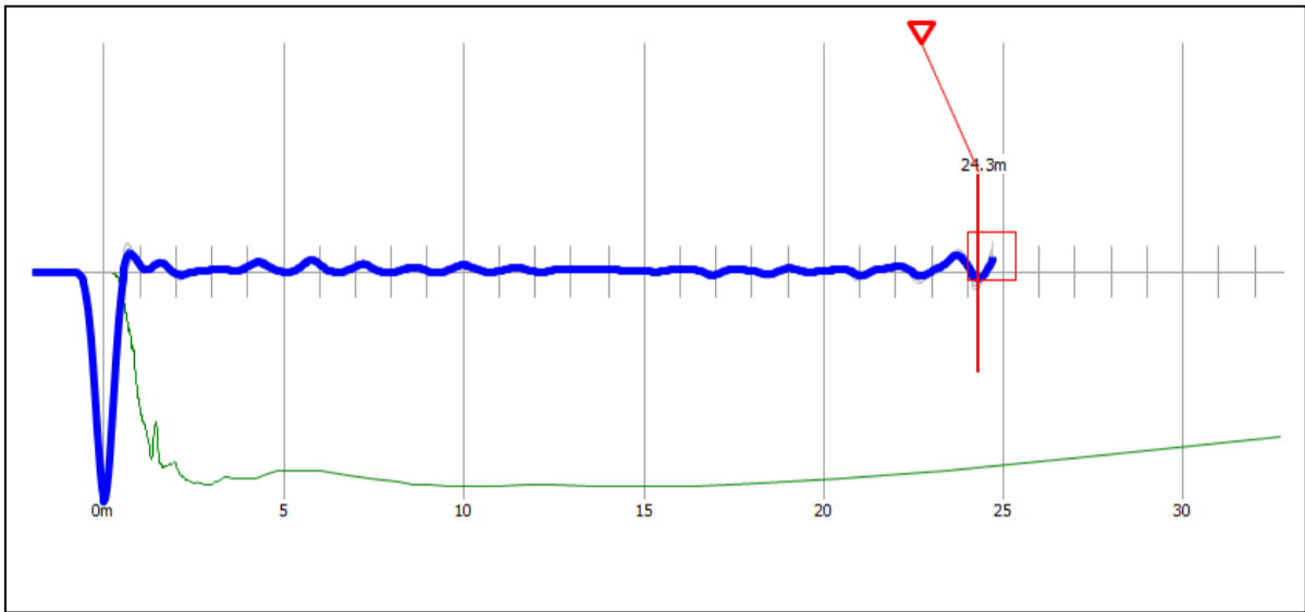
Reflectogram P-186
