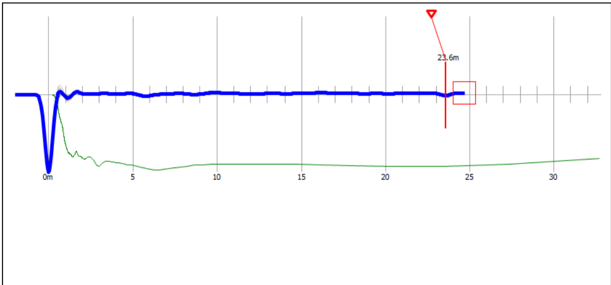
Reflectogram P-117
