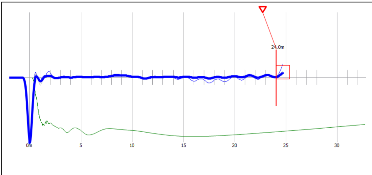
Reflectogram P-136
