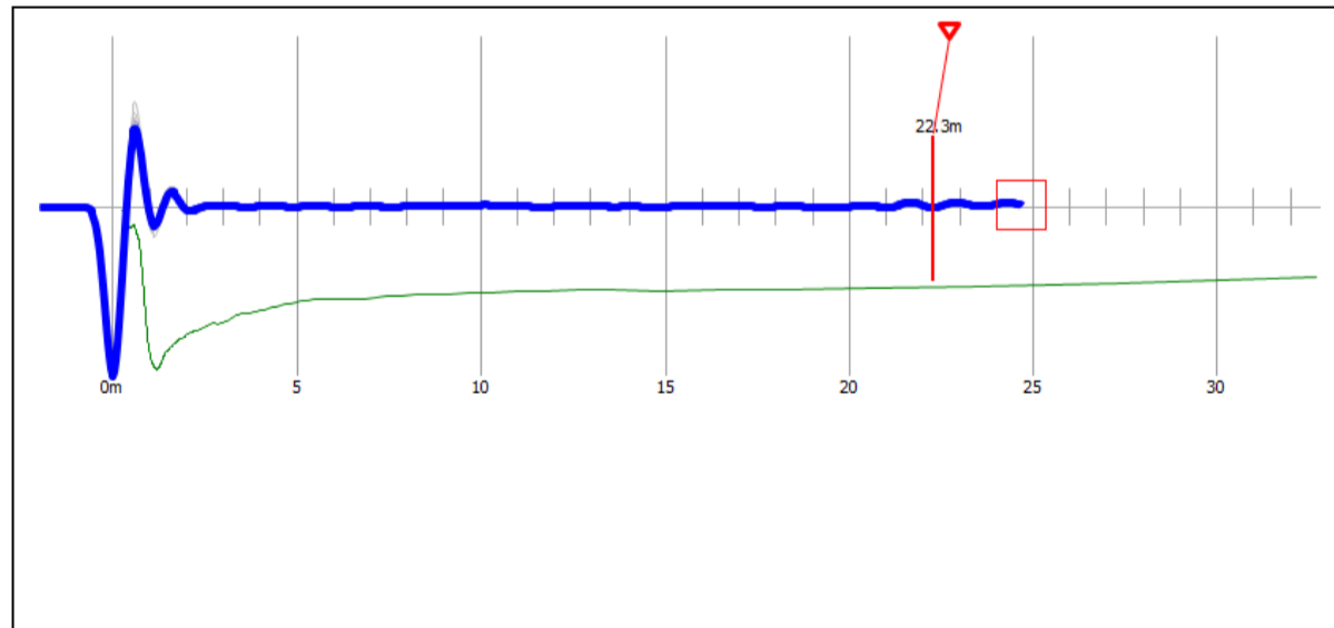
Reflectogram P-90
