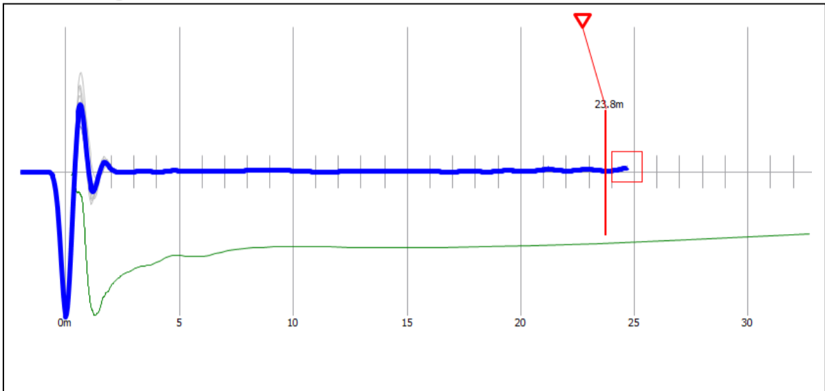
Reflectogram P-298
