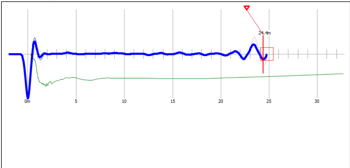
Reflectogram P-18
