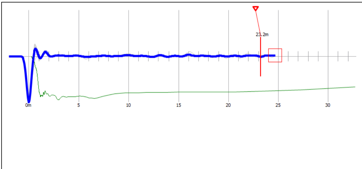
Reflectogram P-109
