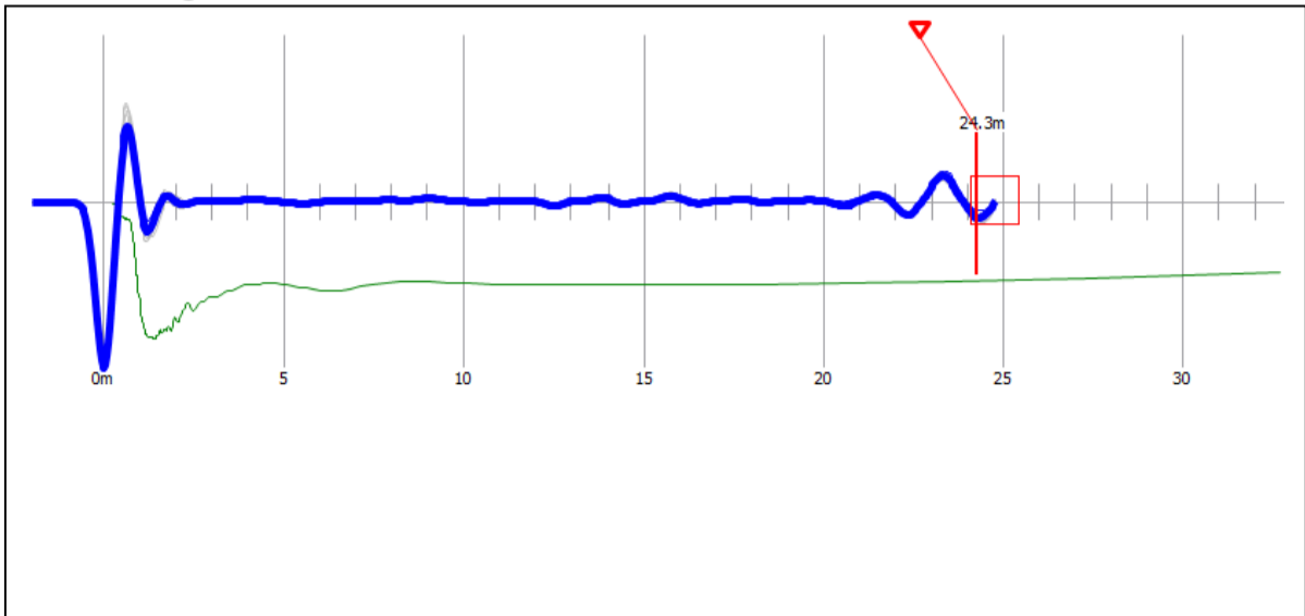
Reflectogram P-8
