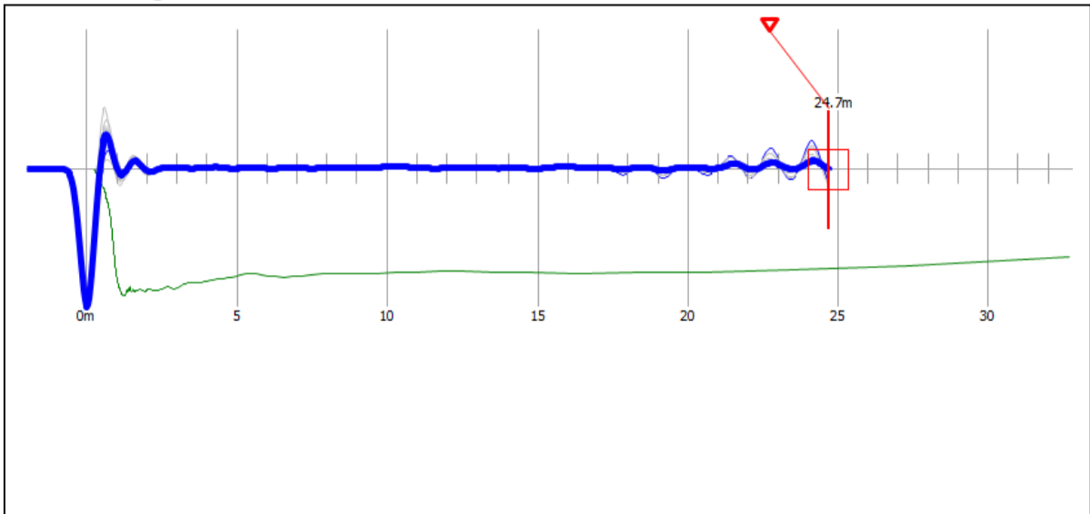
Reflectogram P-78
