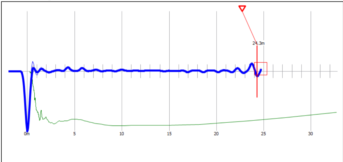
Reflectogram P-240
