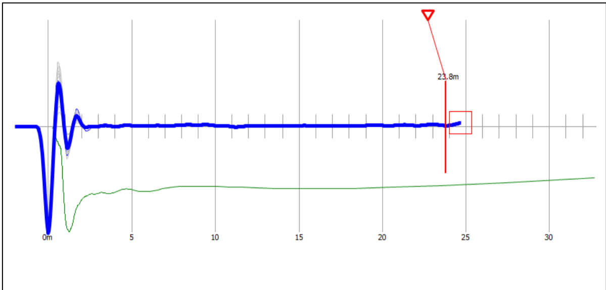
Reflectogram P-310
